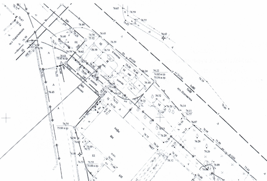
Схема розташування тимчасової споруди по вул. Полтавській в місті Могилеві-Подільському, що підлягає демонтажу.
